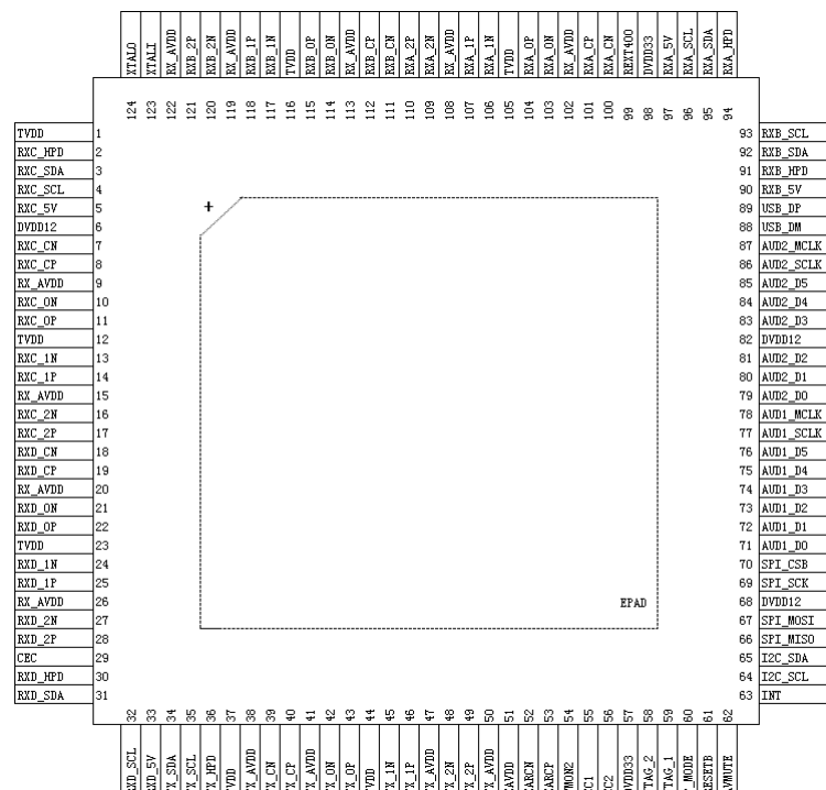
GSV6715 QFN124 Pin Diagram
