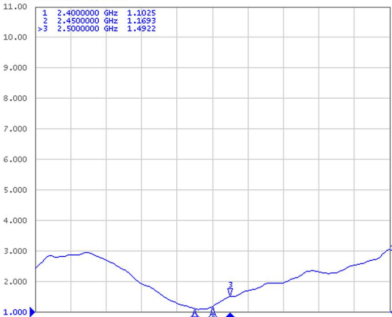
▶ S22 SWR 1.000/ Ref 1.000
