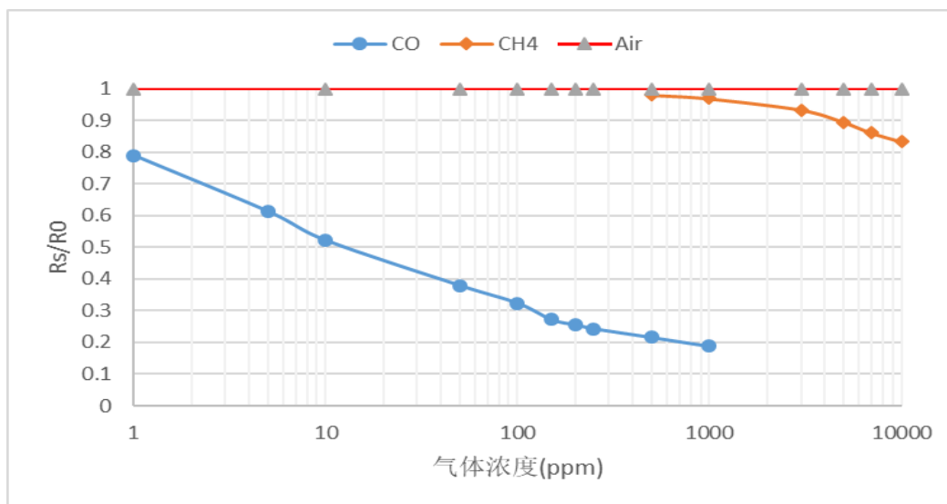
传感器典型的灵敏度对数特性曲线
