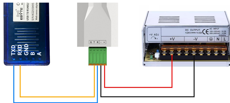
RS232 连接
