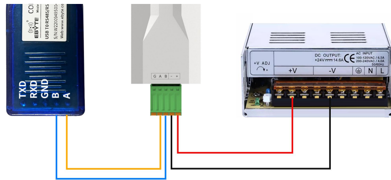
RS485 连接
