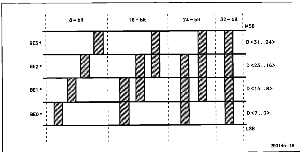
Figure 5-4. Byte Lanes
