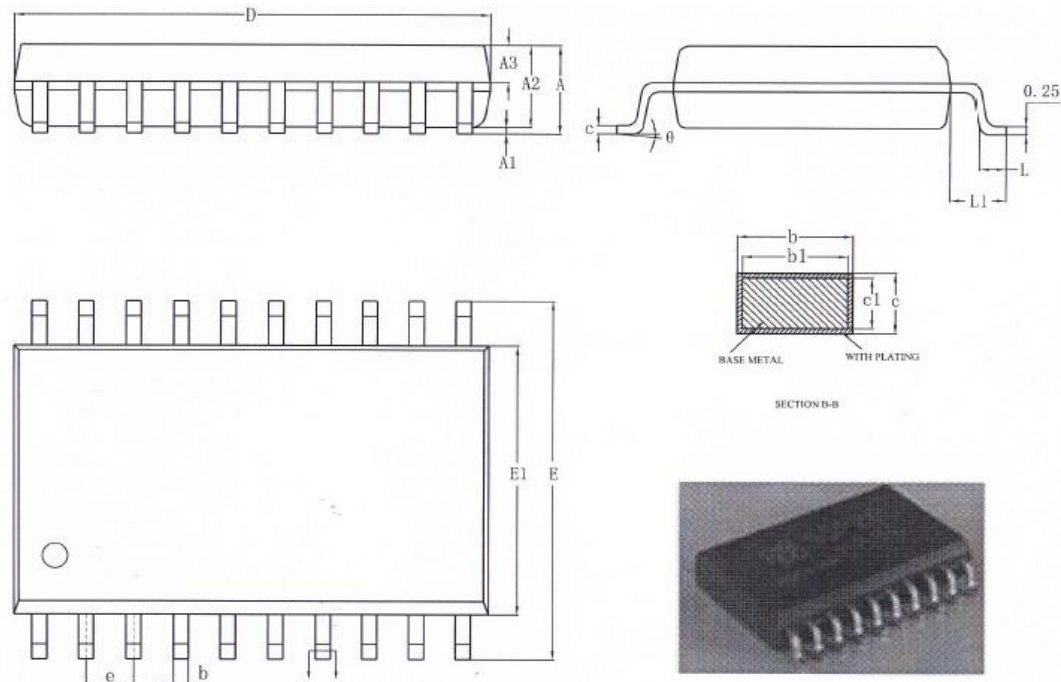
SOP20 package
