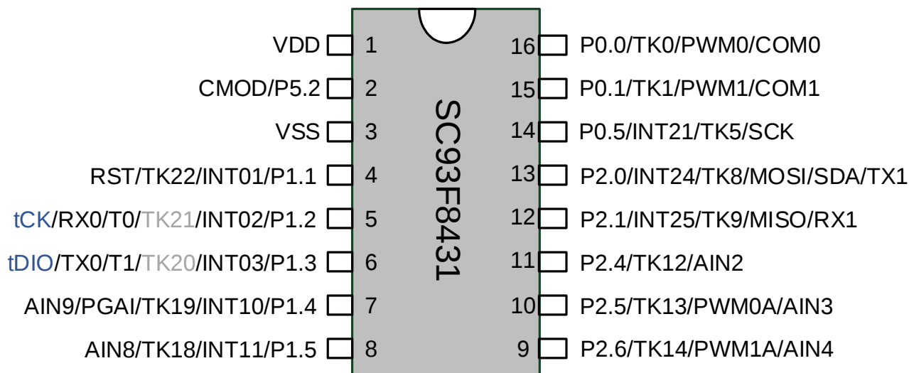
SC93F8431 管脚配置图
