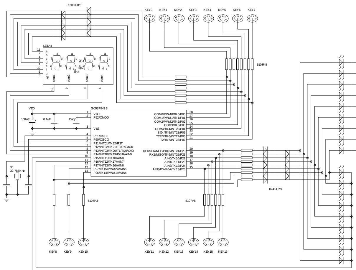
SC93F8433 Touch Key 应用电路：Touch Key 与 LED 共用
