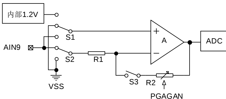
PGA 模式配置图
