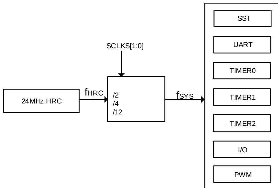
SC93F843X 内部时钟关系
