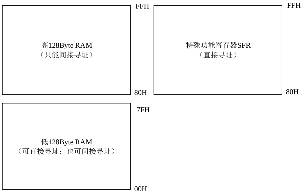
内部 256Byte RAM 结构图
