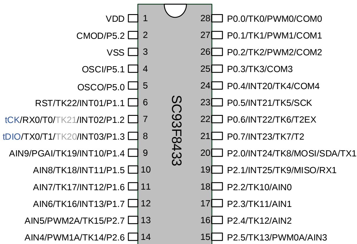
SC93F8433 管脚配置图
