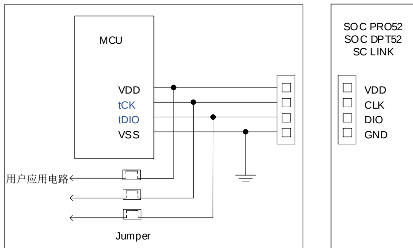
ICP 模式 Flash Writer 编程连接示意图
