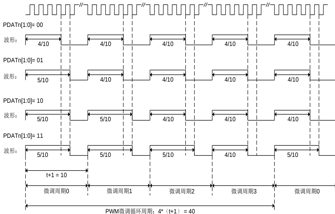
8+2 位 PWM 微调控制示意图
