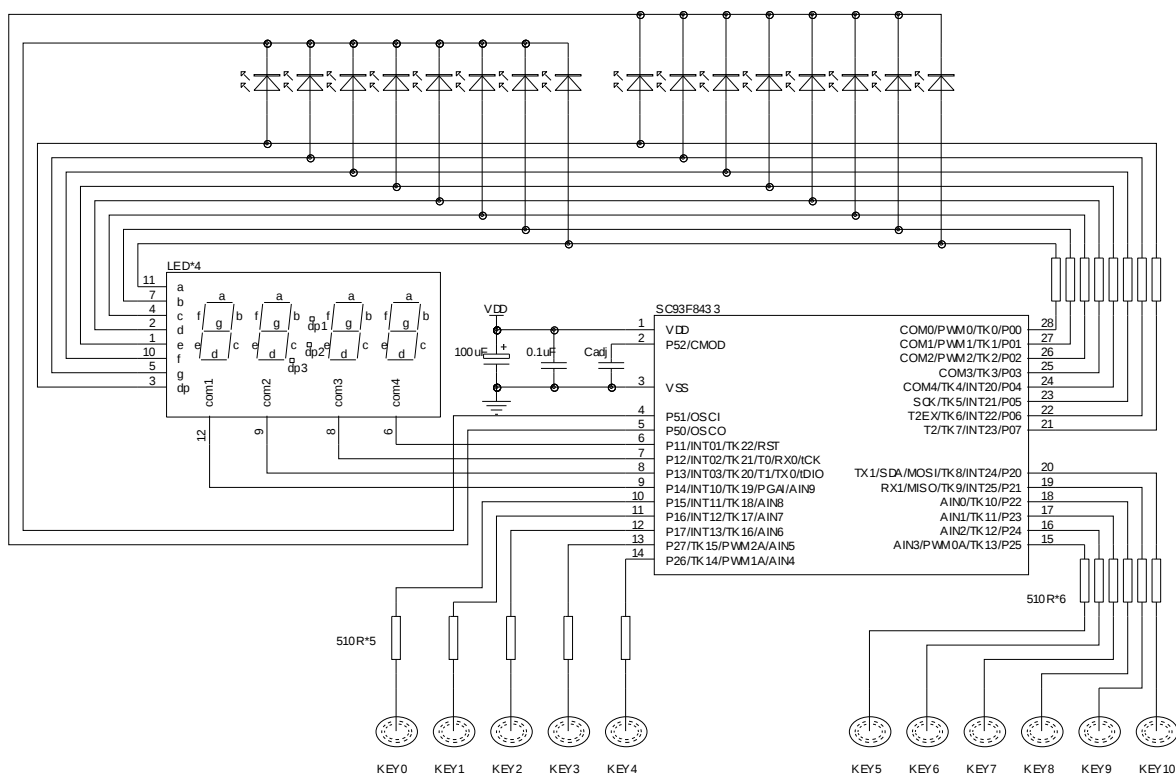
SC93F8433 Touch Key 应用电路图
