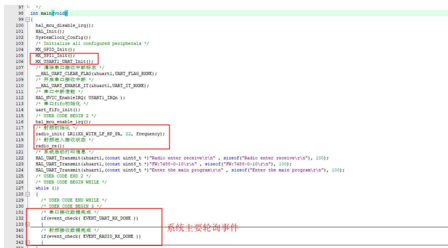
④E80_DEMO main 函数入口;
