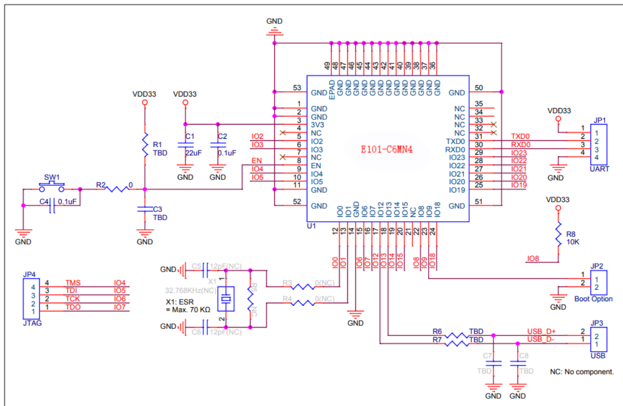
图表 2-3 推荐原理图
