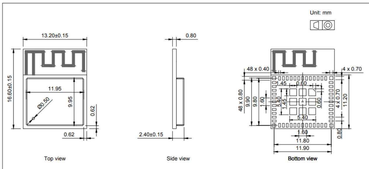
图表 2-4 模组尺寸
