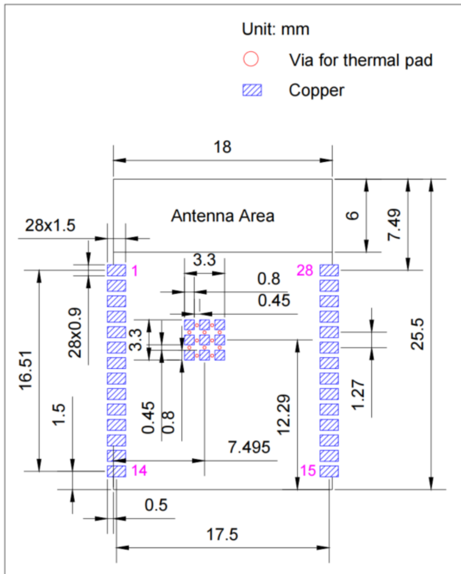
图表 2-6 PCB 封装
