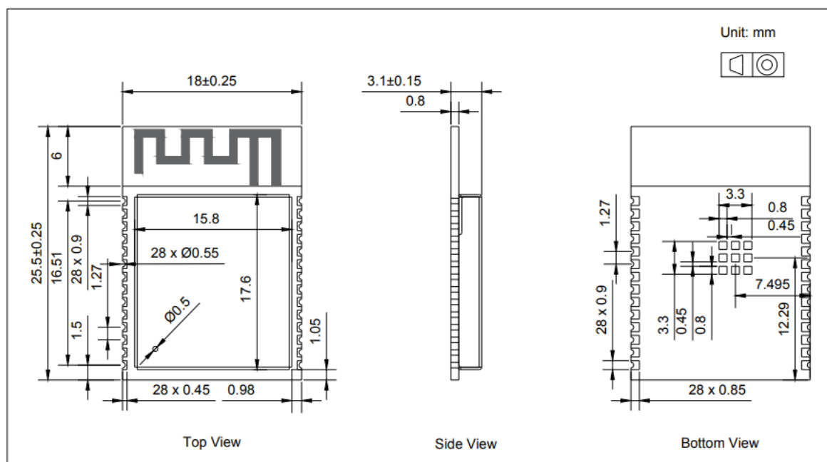
图表 2-3 模组尺寸
