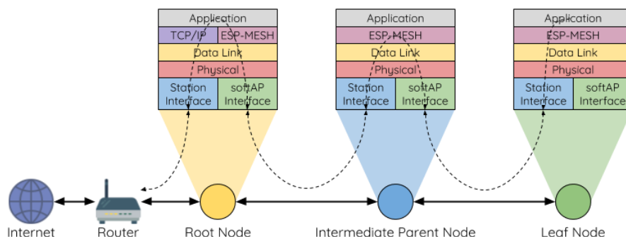
图表 0-2 MESH 数据流
