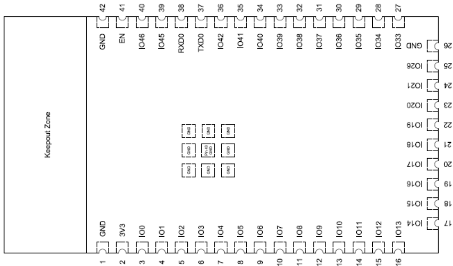
图表 0-1 管脚布局图（顶视图）
