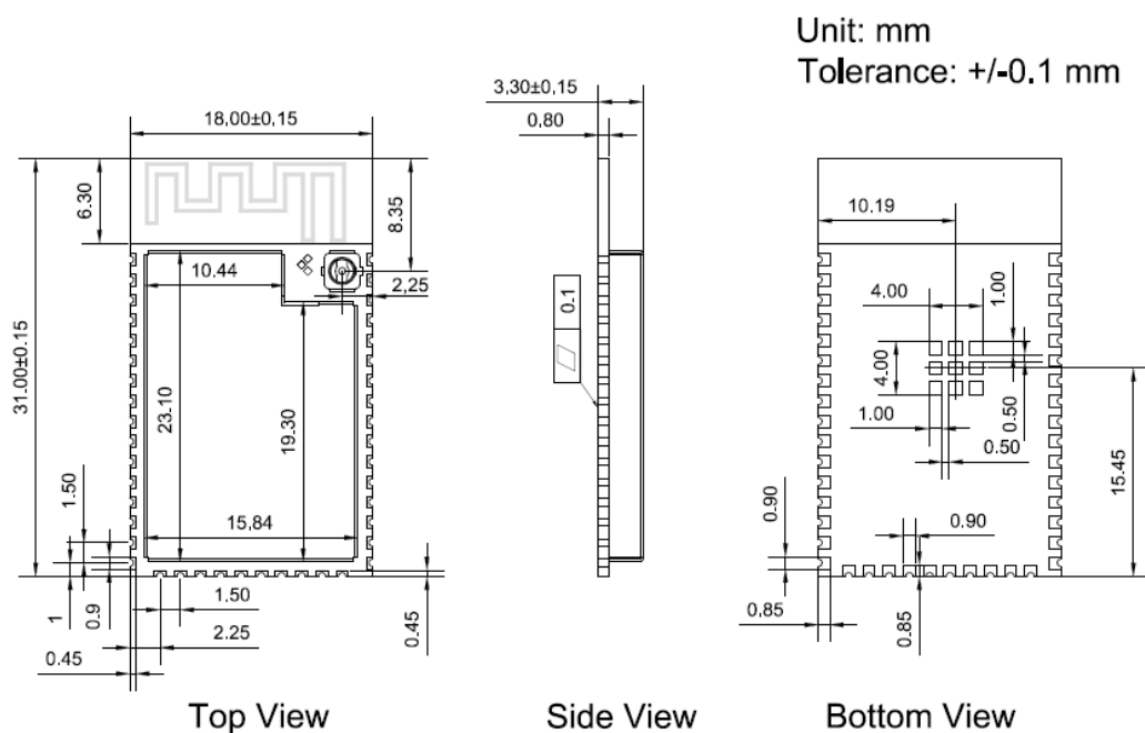
图表 0-4 模組尺寸
