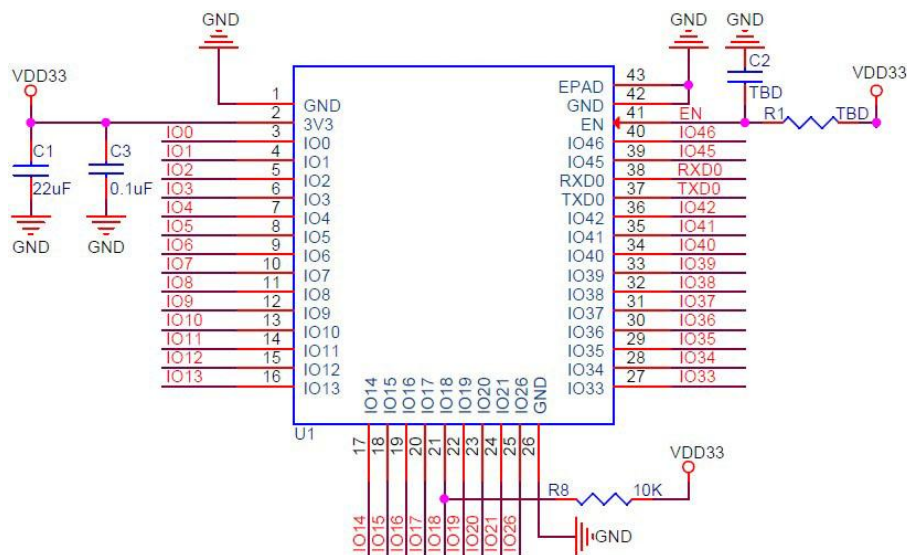
图表 0-3 最小原理图
