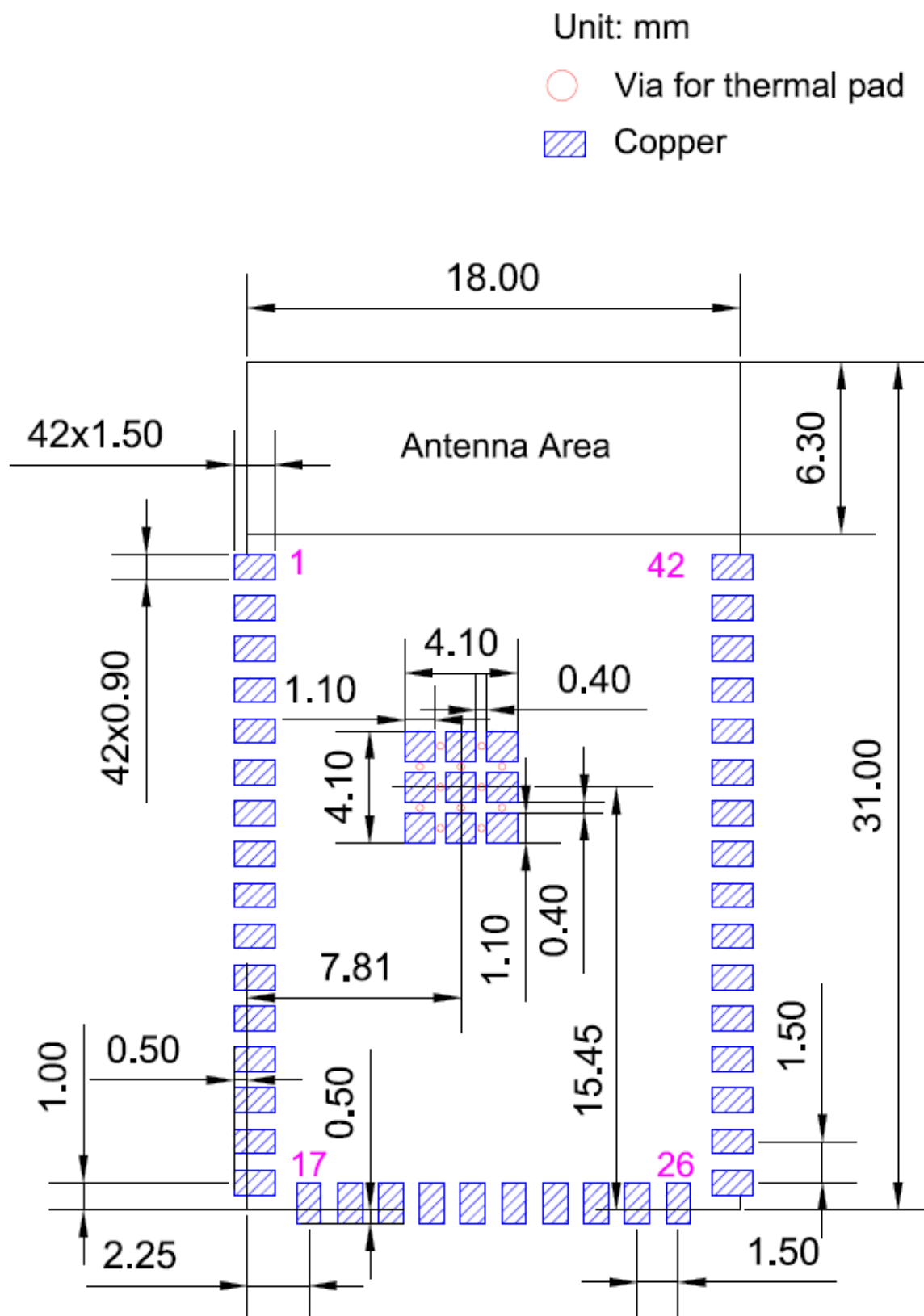
图表 0-5 PCB 封装
