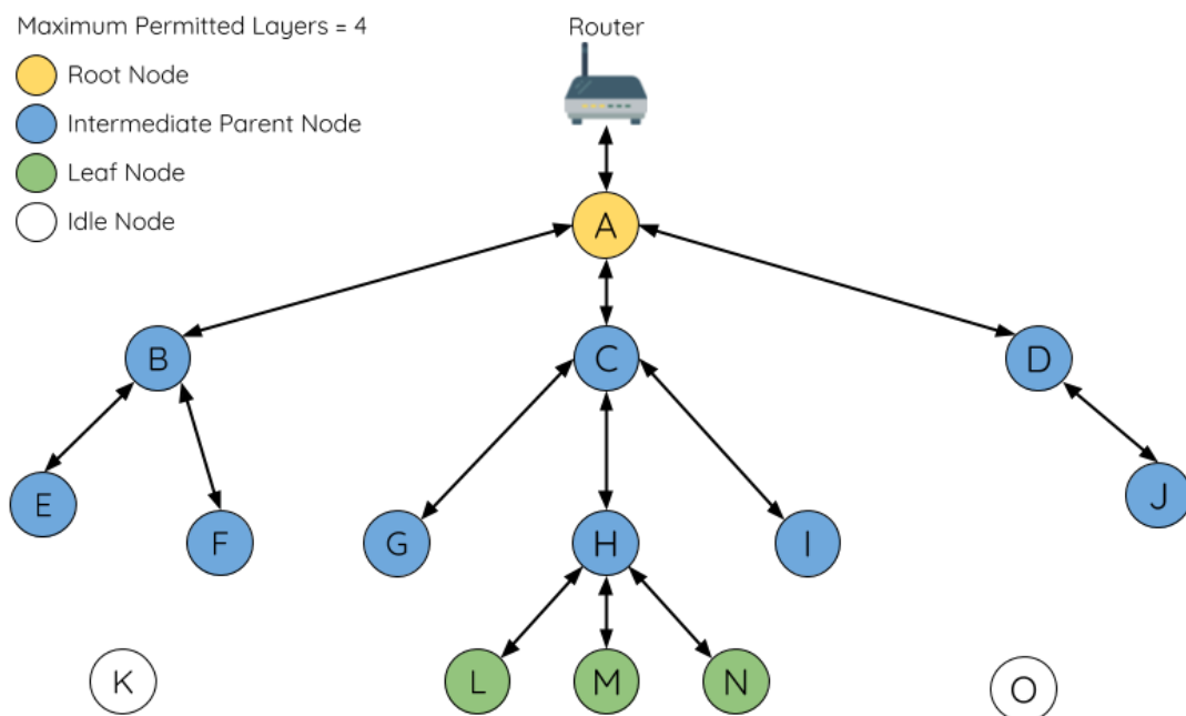
图表 0-1 MESH 网络拓扑图
