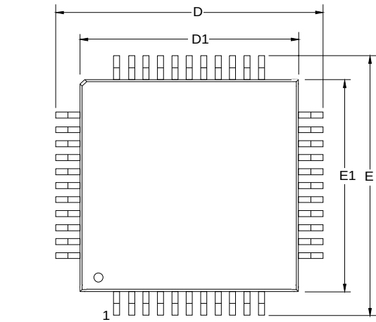
44 PIN TQFP
