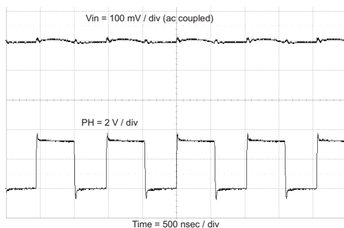
INPUT RIPPLE, 0 A
