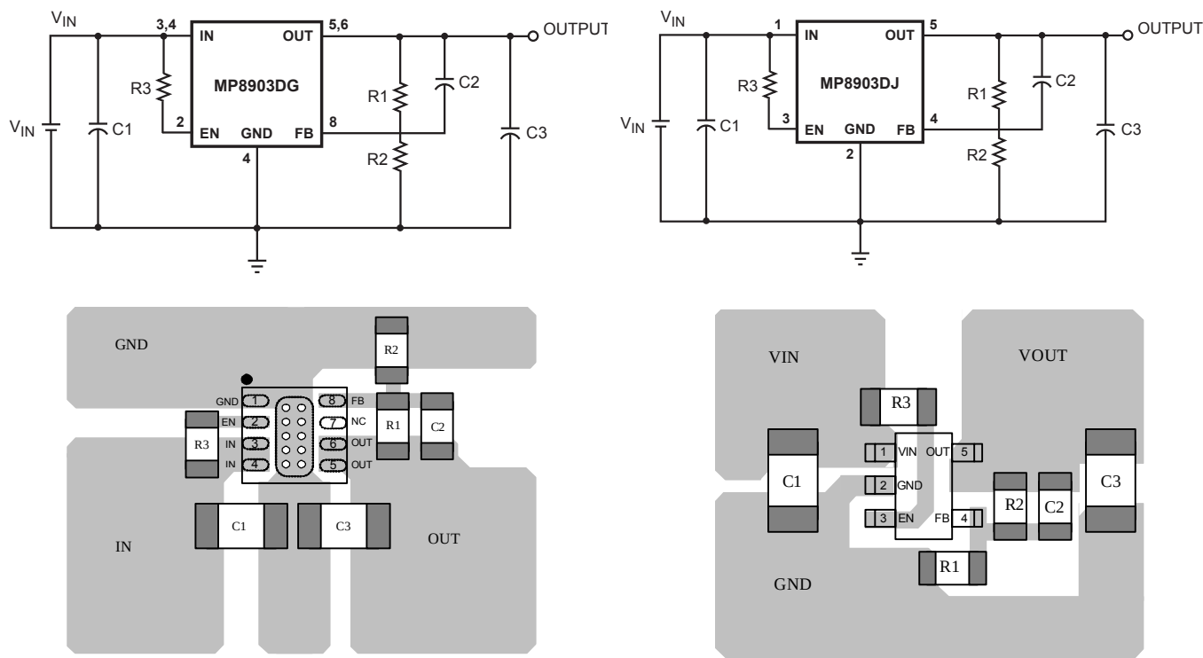
Top Layer
