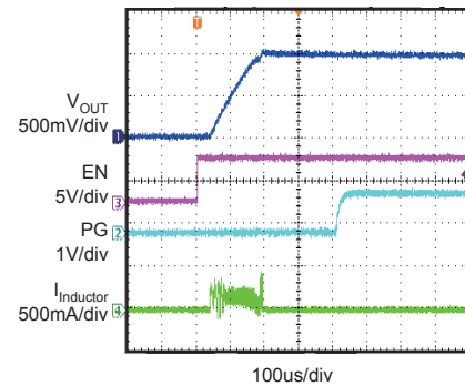
Enable Startup for ASYN Mode
