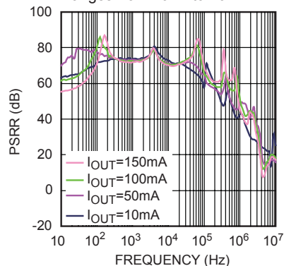
PSRR
