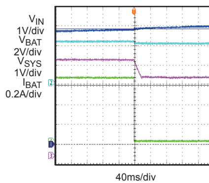
Input OVP
